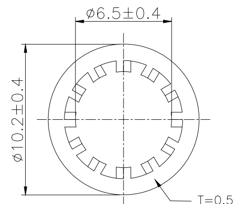
Gasket
